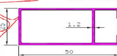
20746 0.529 kg/m
