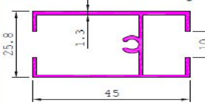
20746 0.529 kg/m
