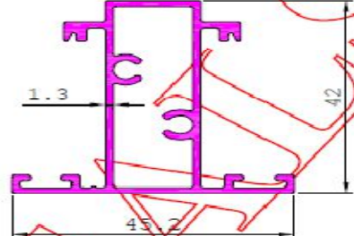
S3169 0.709 kg/m
