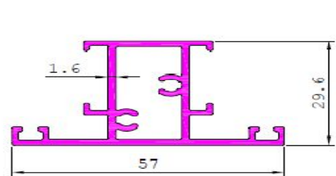
S3306 0.768 kg/m
