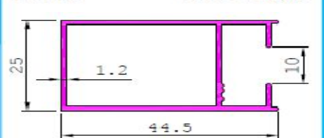
20543 0.669 kg/m
